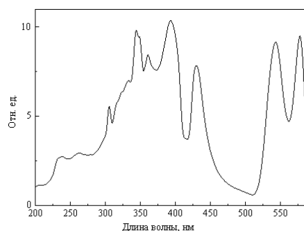
Рис. 4. Отношение спектра поглощения ликвора больного и усредненного спектра поглощения ликвора группы здоровых людей
