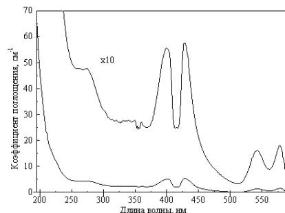
Рис. 1. Спектр поглощения ликвора больного и длинноволновая часть спектра, растянутая в 10 раз по коэффициенту поглощения.
