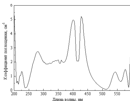
Рис. 2. Спектр поглощения ликвора больного за вычетом коротковолновой полосы
