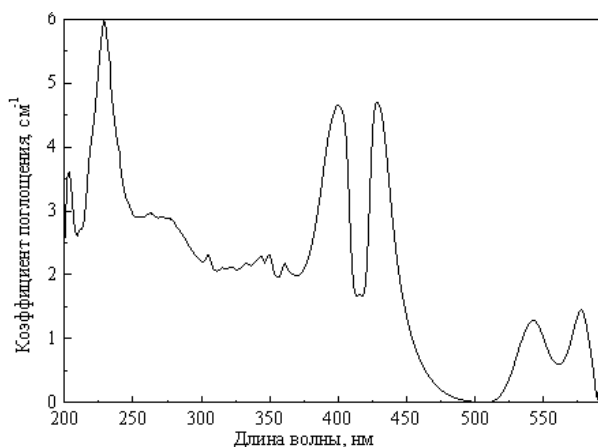
Рис. 3. Разность спектра поглощения ликвора больного и усредненного спектра группы здоровых людей.
